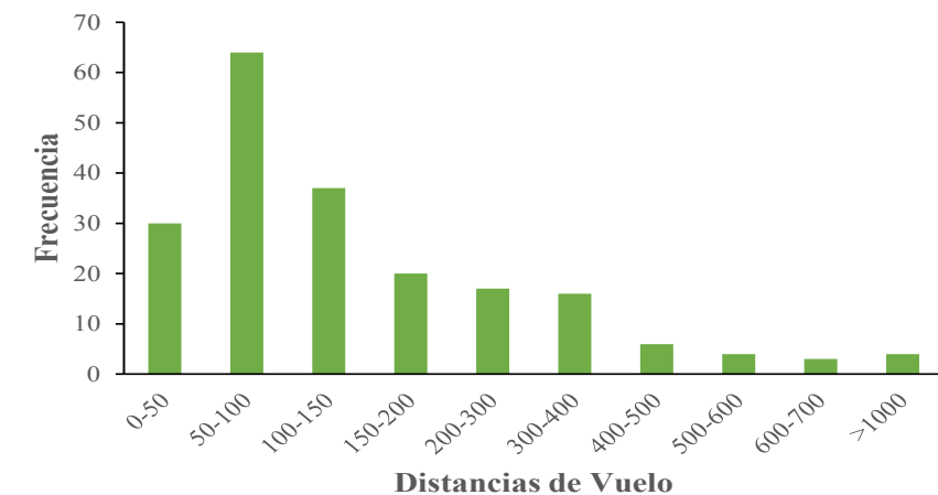
Figura 9. Frecuencias de distancias de vuelo del tercer grupo de pericos monitoreado.
