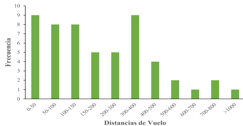
Figura 5. Frecuencia de distancias de vuelo en el primer grupo de pericos monitoreados.
