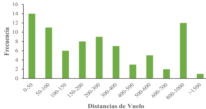
Figura 7. Frecuencias de distancias de vuelo del segundo grupo de pericos monitoreado.
