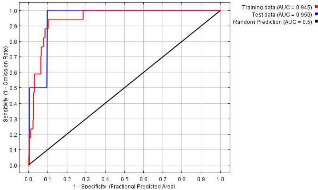
Figura 12. Prueba AUC para la validación del modelo de distribución del Pyrrhura orcesi .
