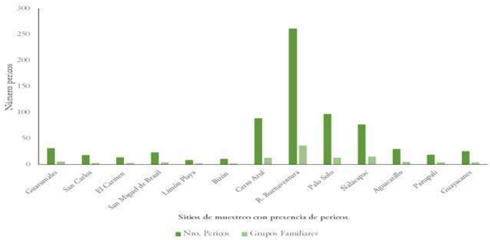
Figura 2. Abundancia del perico de El Oro Pyrrhura orcesi en las localidades estudiadas con respecto a la Reserva Buenaventura.
